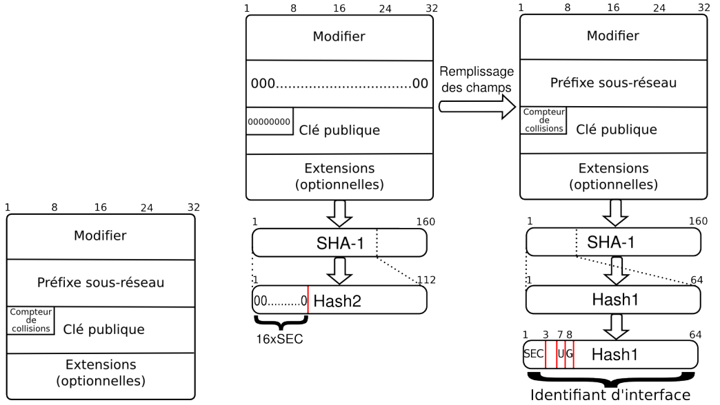
Figure 3: Structure de données paramètres CGA
