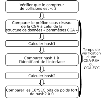
Figure 6: Algorithme de vérification d'une CGA
